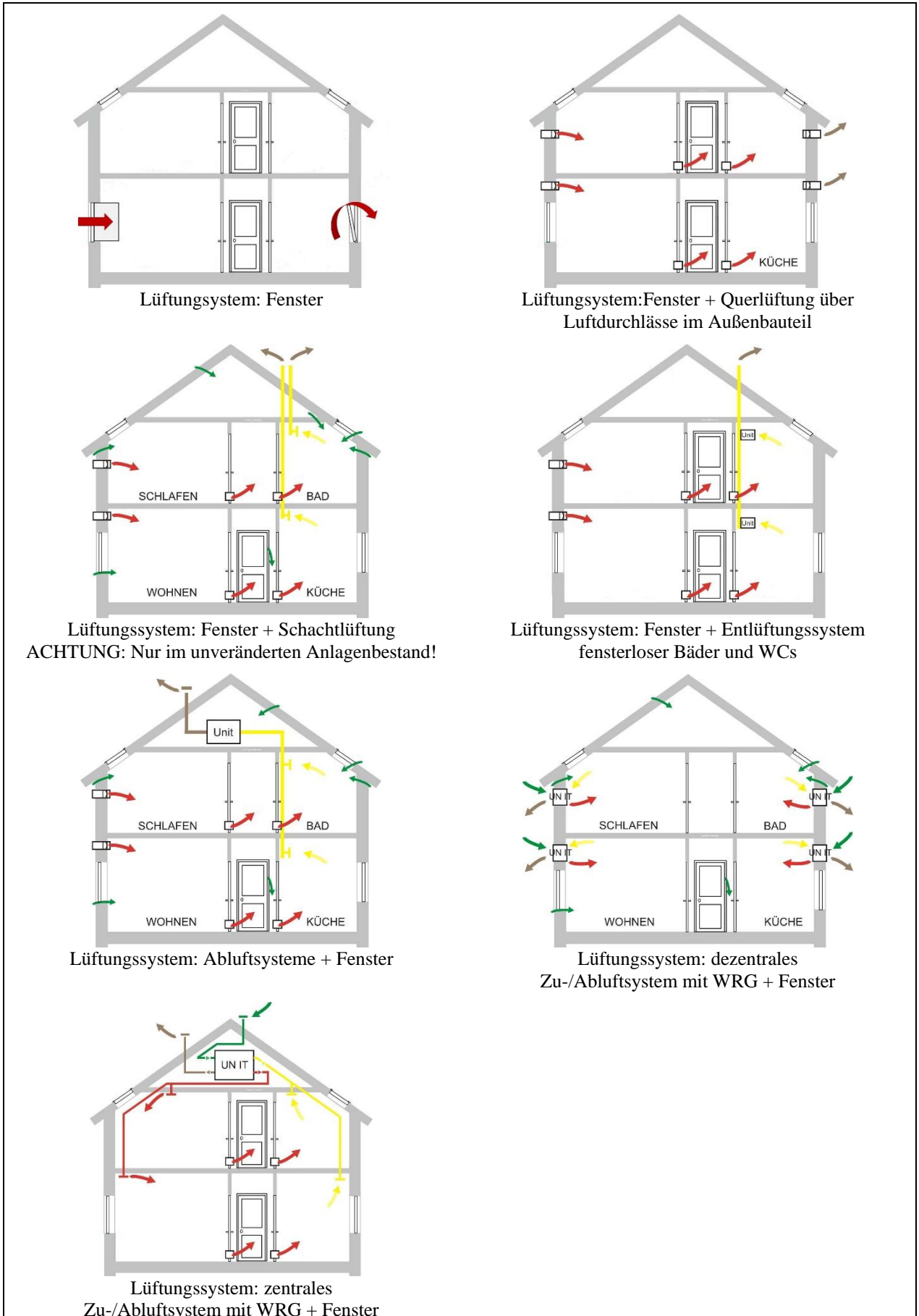
Übersicht der behandelten Lüftungssysteme, Quelle: Berhorst / Reiners
